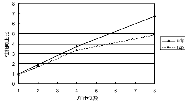
図 5:マンデルブロー集合による評価
