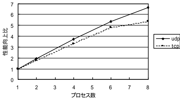
図 3:多体問題の性能評価 (星の数1000)
